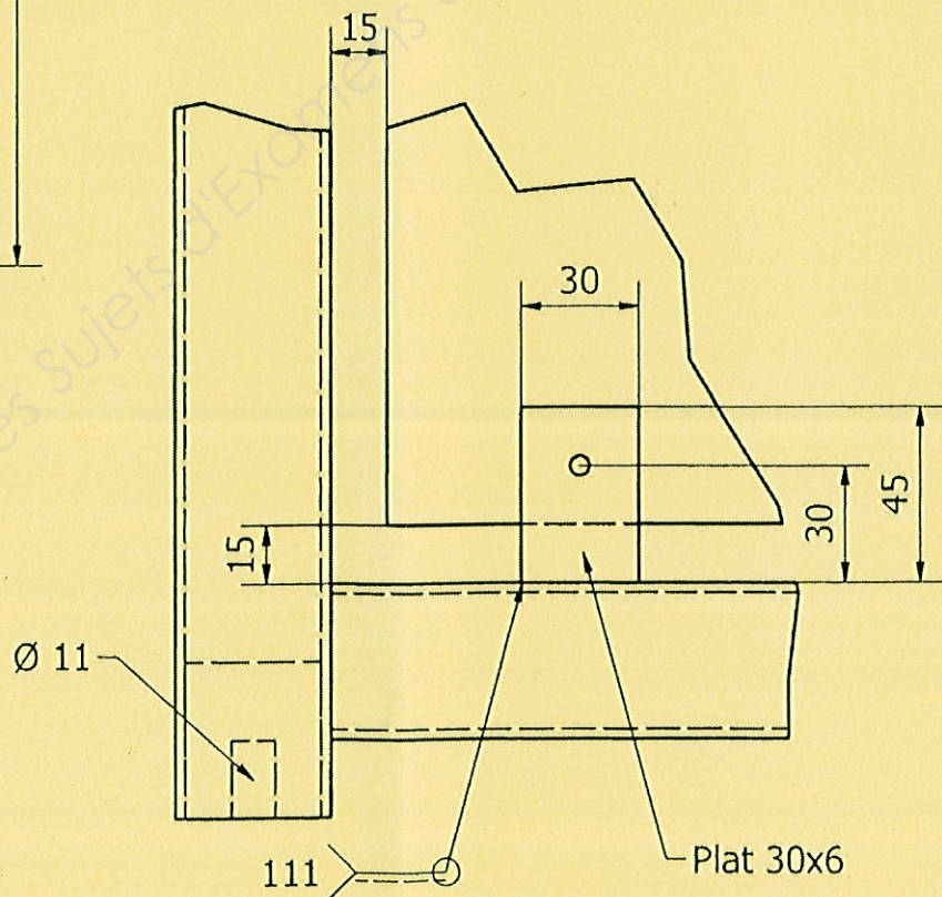
C ( 1 : 2 )
